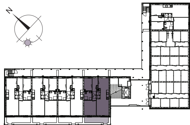
Appartement Bnr. 127 | Begane grond
